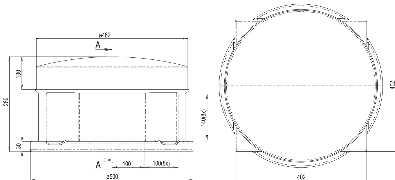
Rysunek techniczny
