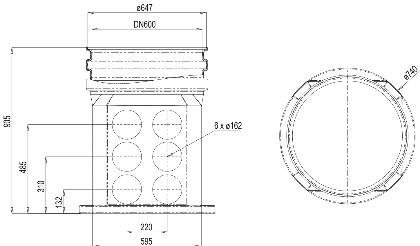
Rysunek techniczny
